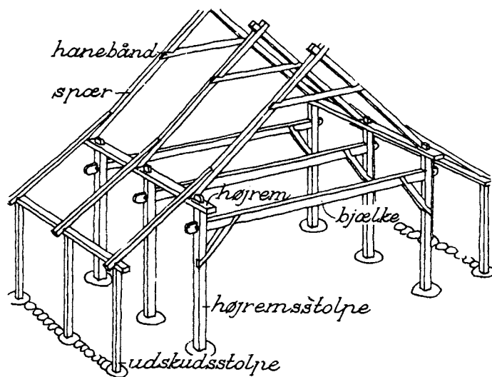
Udskuds- eller højremskonstruktion af nyere type med korrespondance mellem højrem- og vægstolper. - Fig.4.
